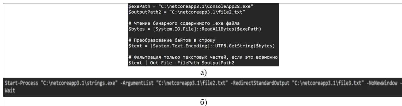
Рисунок 1. Дизассемблирование EXE-файла
